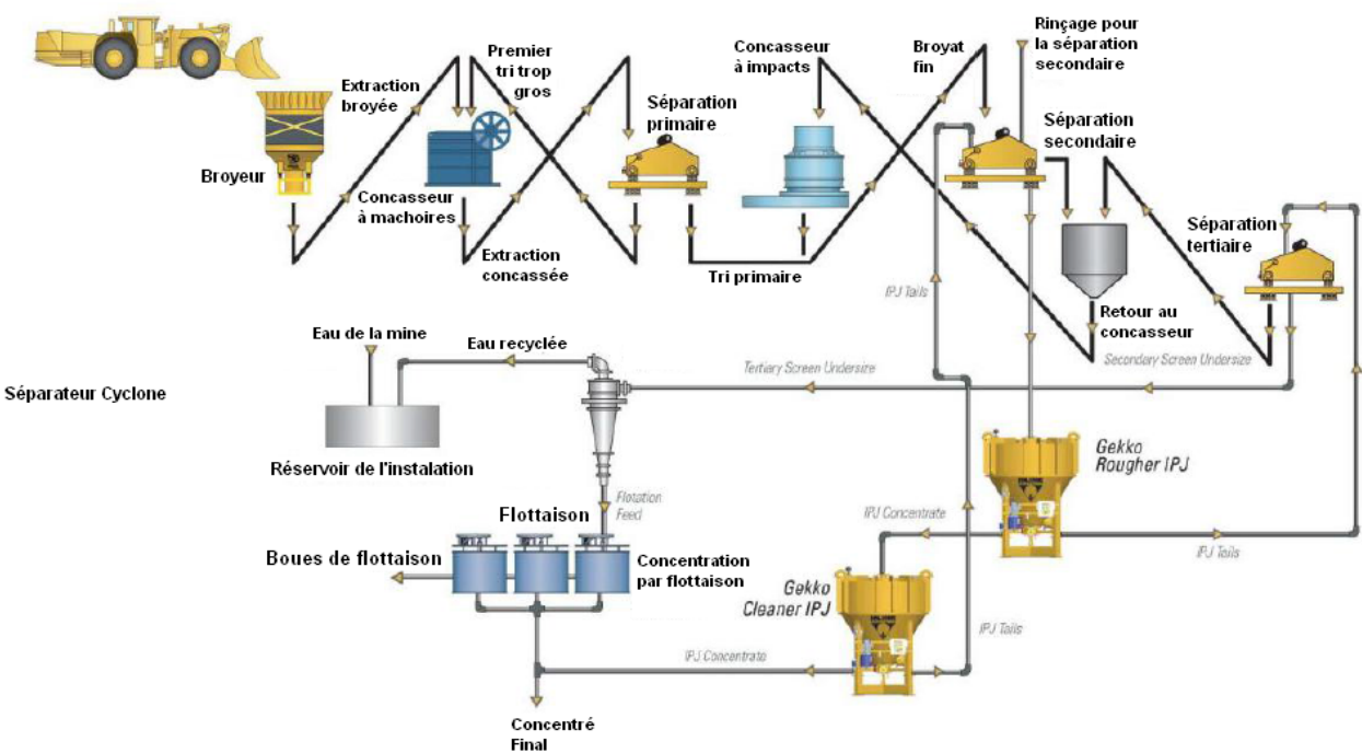
Schéma de l'installation industrielle mobile Gekko Python
